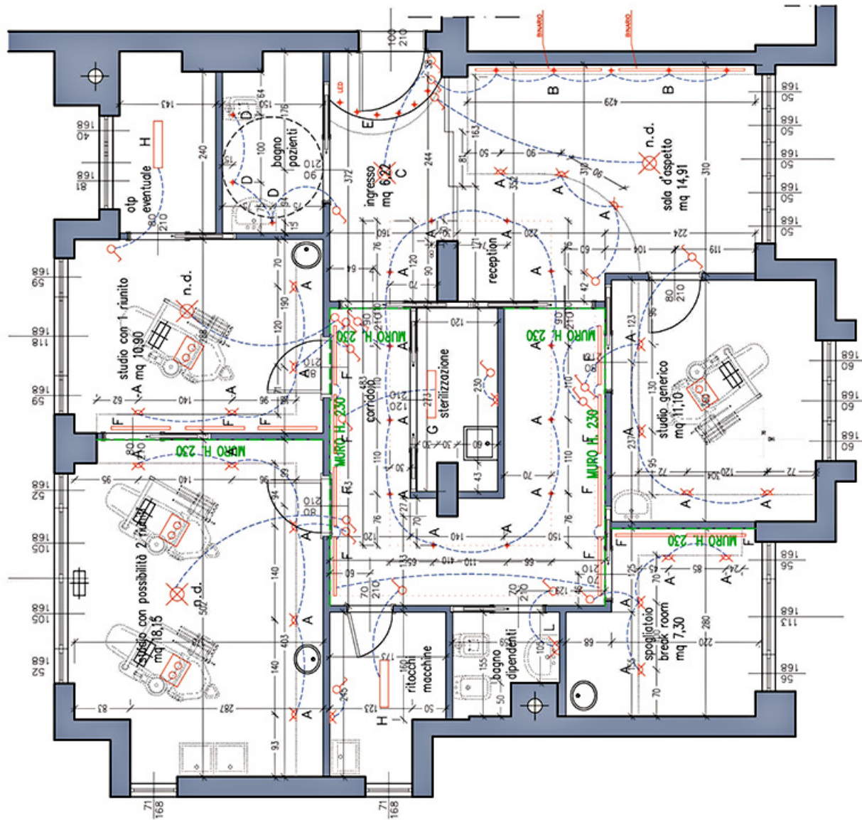
Impianto illuminotecnico
